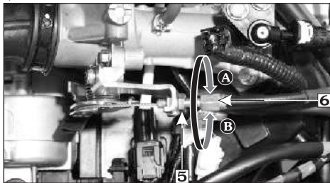
(5) Contratuercas (6) Tuerca de ajuste (A) Disminuir el juego libre (B) Aumentar el juego libre
