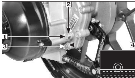
(1) Perno de control (3) Perno de drenaje
