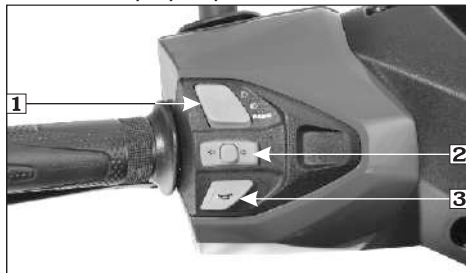
(1) Regulador intensidad/Interruptor de paso (2) Interruptor luz de giro (3) Interruptor de la bocina
